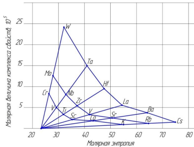
Рисунок 1. Диаграмма теплофизических свойств K_{\mu} - S_{\mu} [4].
