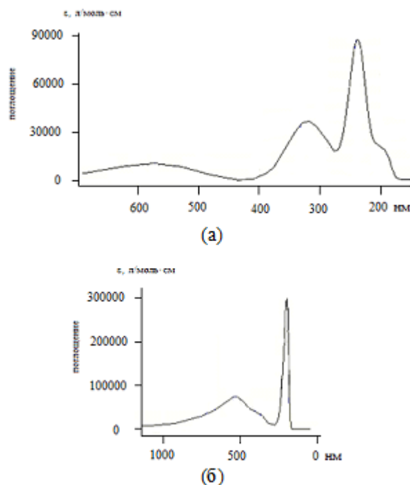
Рисунок 3. Электронные спектры поглощения графенового листа без (а) и полностью легированного (б) атомами Si.
