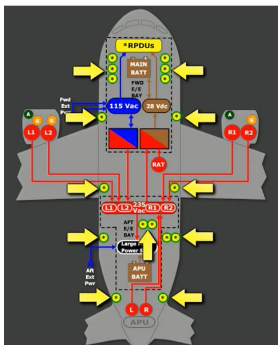
Рисунок 2. Система распределения электроэнергии Boeing-787.
