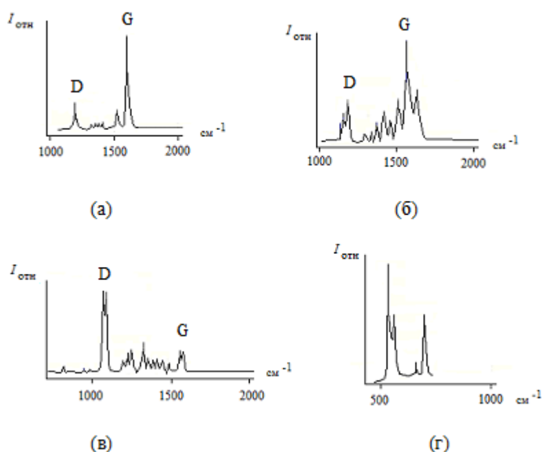
Рисунок 2. Спектры КР графена (а), легированного 1-м (б), 6-ю (в) и полностью атомами (г) Si.
