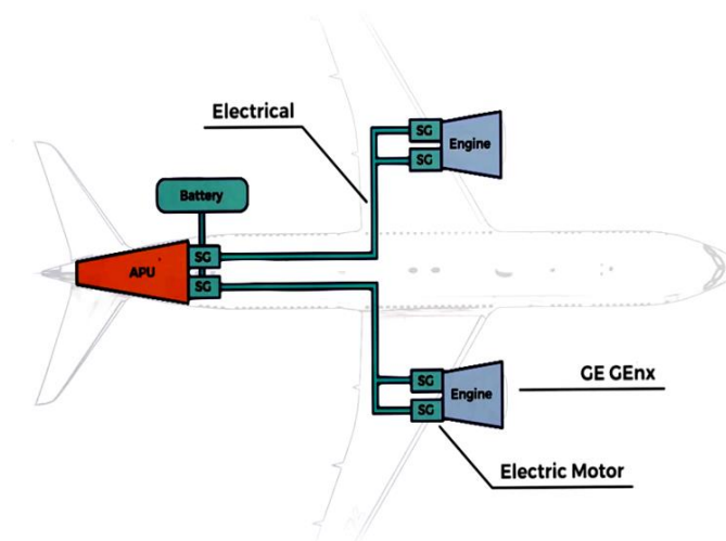
Рисунок 1. Схема расположения генераторов энергии на Boeing-787.
