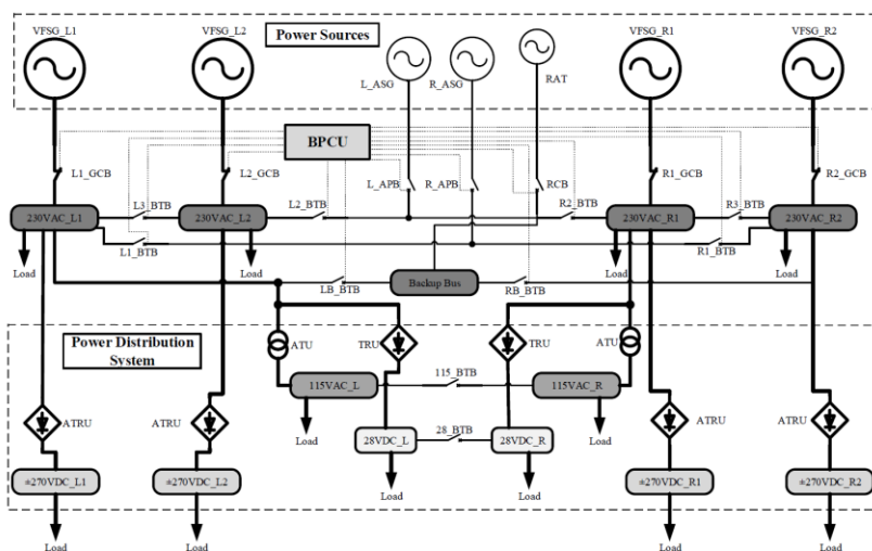
Рисунок 1. Электрическая схема Boeing-787.
