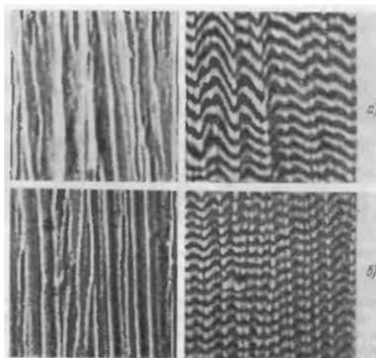
Рисунок 3. Мартенситный рельеф: а-закалка без поля; б-закалка в магнитном поле.
