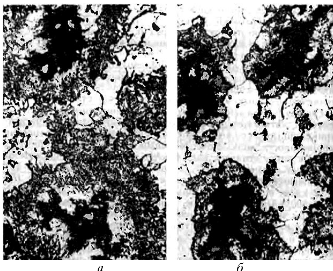
Рисунок 1. Микроструктура ферритного ковкого чугуна после закалки от 900°C при нагреве т.в.ч. без поля (а) и в магнитном поле напряженностью 1,44 МА/м (б), \times 500
