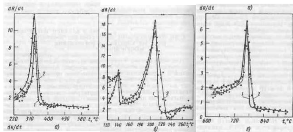
Рисунок 1. Температурные зависимости dR/dt для стали 30ХГСА (а), 0Н18К9М5Т (б), и технического железа (в)
