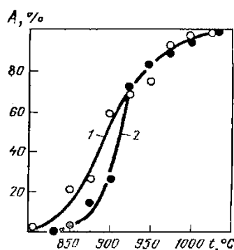
Рисунок 3. Аустенитизация ферритного ковкого чугуна: 1-нагрев без поля; 2-нагрев в магнитном поле напряженностью 1,44 МА/м
