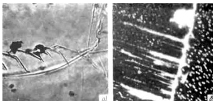
Рисунок 2. Рост аустенита по сдвиговому механизму (рельеф) от малоугловой (а) и высокоугловой границы (б, темное поле), сталь 30ХГСА, нагрев в вакууме, \times 650
