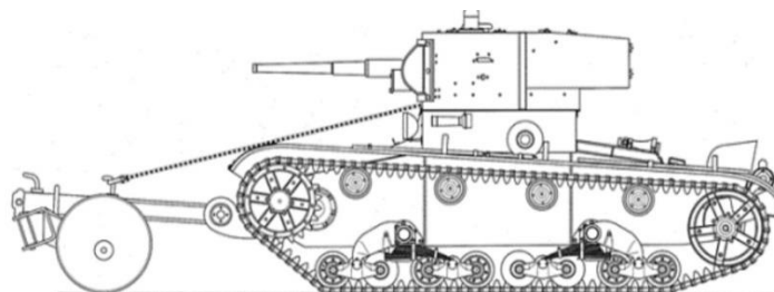
Рисунок 2. Минный трал, установленный на танке Т-26 [5].
