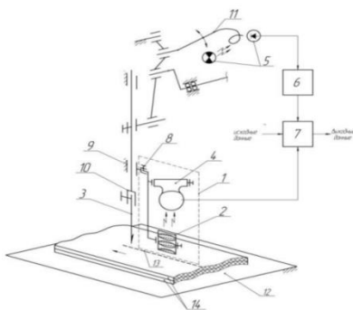
Рисунок 1. Схема устройства для оценки повреждаемости нитей материалов при выполнении швейных строчек.
